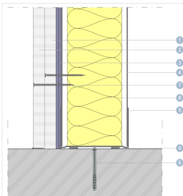
VarioShield Plus
